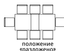
Стол обеденный «Моника» (с механизмом) П4.646.4.02-Р: L1600/2000xВ900xH777 Стол обеденный «Моника» (с механизмом) П4.646.4.03-Р: L1800/2200xВ1000xH777
