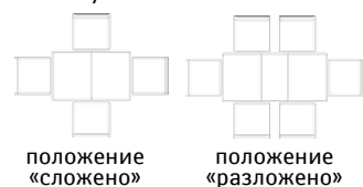
Стол обеденный «Альт» П4.490.4.06: L1080/1470xВ670xH776
