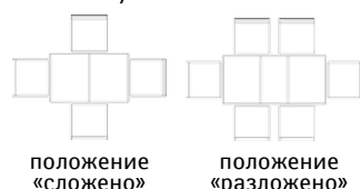
Стол обеденный «Альт» П4.490.4.07: L1330/1720xВ720xH776
