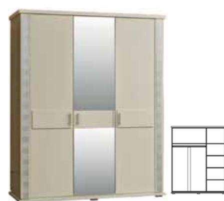
Шкаф для одежды 3д «Тунис» П6.343.1.01-01: L1752xВ605xH2150
