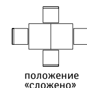
Стол обеденный «Моника» (с механизмом) П4.646.4.07-Р: L1100/1500xВ700xH777 Стол обеденный «Моника» (с механизмом) П4.646.4.00-Р: L1200/1600xВ800xH777 Стол обеденный «Моника» (с механизмом) П4.646.4.01-Р: L1400/1800xВ800xH777
