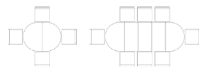
Стол «Милана» П4.265.0.29: L1300/1770/2240/2710xВ1000xH778
