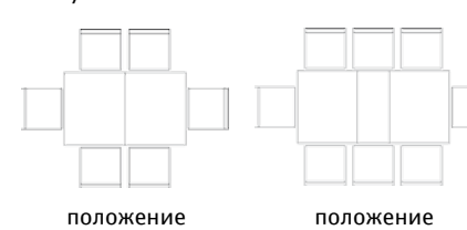
Стол обеденный «Альт» П6.490.4.22: L1500/1900xВ900xH776 Стол обеденный «Альт» П6.490.4.23: L1100/1490xВ900xH776
